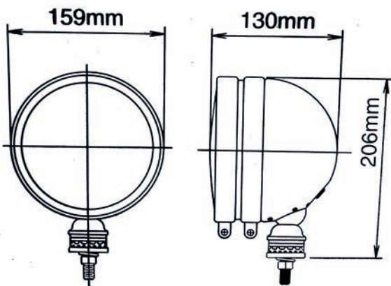
FARO LUNGA PORTATA Ø 16 / 100w / Singolo Nero : PHI01N
